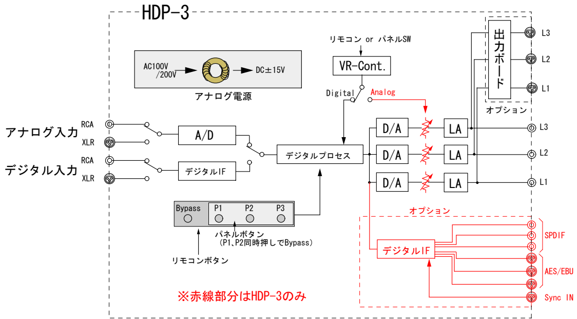
HDP-3 の内部構成
