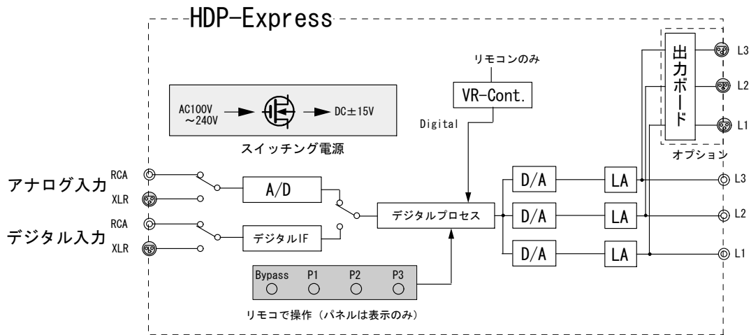
HDP-Express の内部構成
